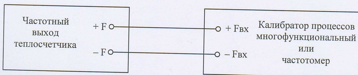
Рисунок Б.2 – Электрическая схема подключения эталонных СИ при поверке активного частотного выхода теплосчетчика.
