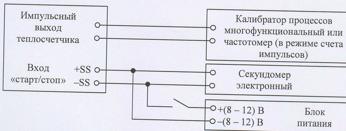
Рисунок Б.3 – Электрическая схема подключения эталонных СИ при поверке импульсного выхода теплосчетчика.
