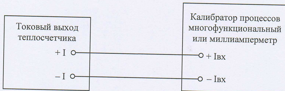
Рисунок Б.1 – Электрическая схема подключения эталонного СИ при поверке токового выхода теплосчетчика
