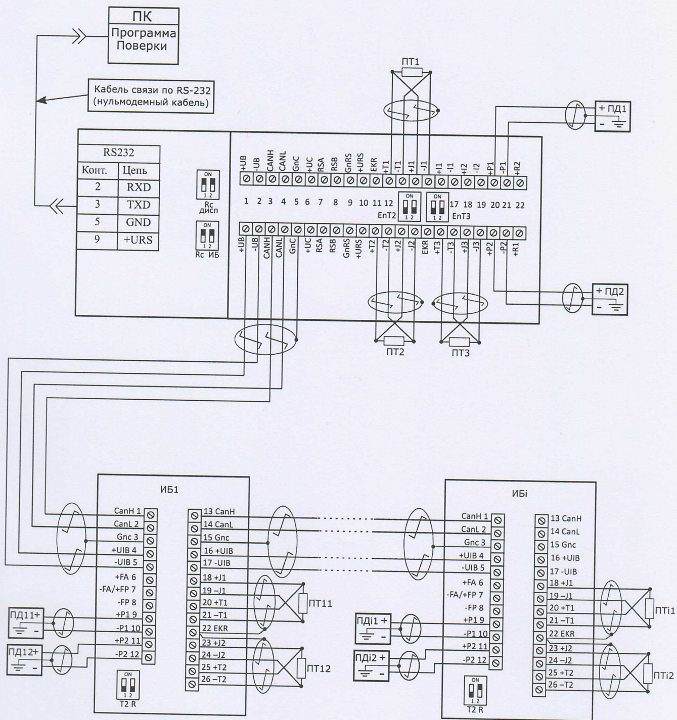
Рисунок А.4 – Электрическая схема подключения многопоточного теплосчетчика с TeRoss-ИБ, имеющим цифровой выход
